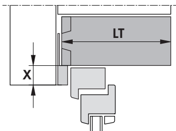
Obr. B – Omietací plech do ostenia / nadpražia (4)
